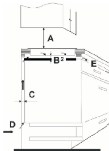
Schéma II Sur les tiroirs et meubles B2= sans source de chaleur
